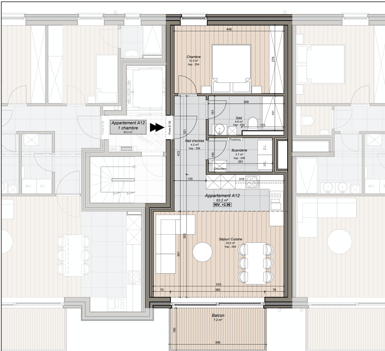
Appartement A12 - Echelle : 1/75
